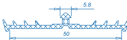
5768 Уплотнение под крышку
