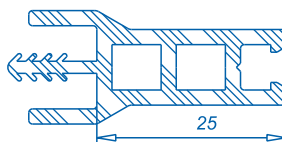
5592 Уплотнение под стеклопакет
