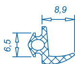
AP001 Уплотнение притвора
