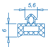
AP-13 Уплотнение под стеклопакет
