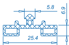
AP003 Уплотнение рамы
