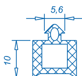
AP-15 Уплотнение под стеклопакет
