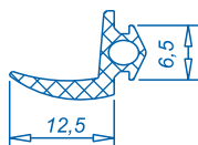
5864 Уплотнение притвора
