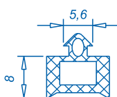
AP-14 Уплотнение под стеклопакет
